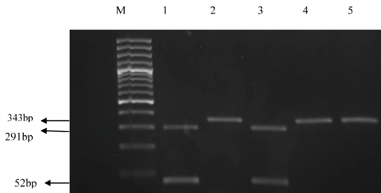
شکل ۱: الکتروفورز محصول PCR-RFLP/اسیتوباکتر بامانی. (M) سایز مارکر ۱۰۰ جفت بازی، ستون ۱) سویه استاندارد پس از هضم آنزیمی، ستون ۲) سویه استاندارد بدون اثر آنزیم، ستون ۳) نمونه مقاوم به کینولون فاقد جهش، ستون های ۴ و ۵) نمونه مقاوم به کینولون دارای جهش.
